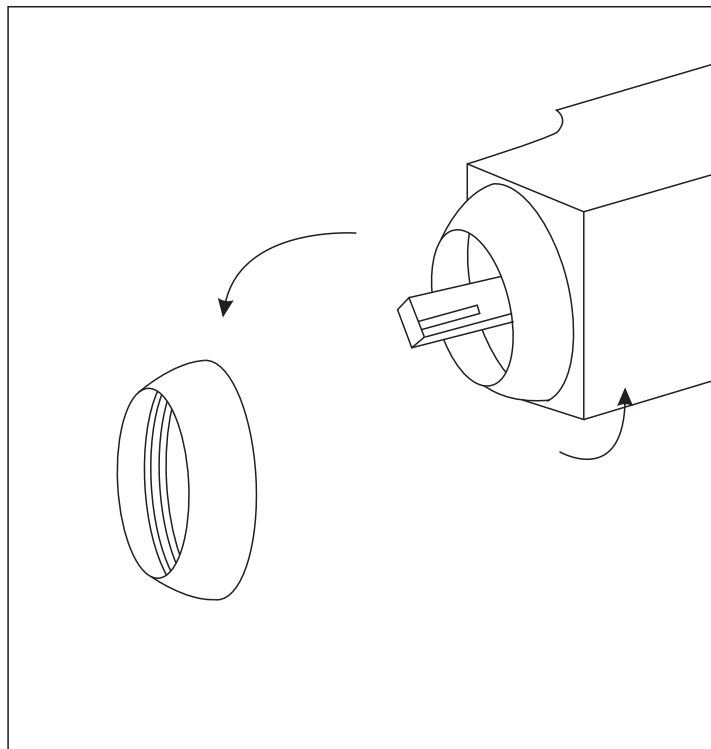
2. Odkręcenie maskownicy
