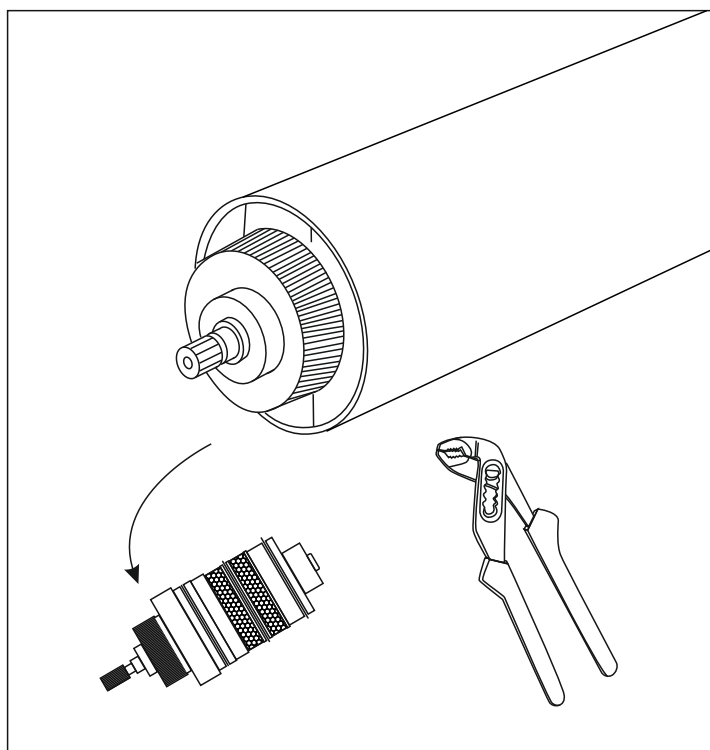
4. Wyjęcie głowicy termostatycznej kluczem nastawnym typu żaba lub kombinerkami
